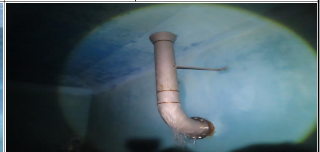
배수지 1지(유입)
